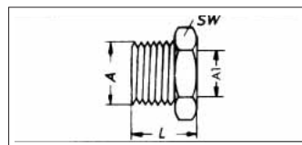
Կրճատ ներագույց
