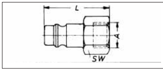
Ներդրվող ծայրափողակ
