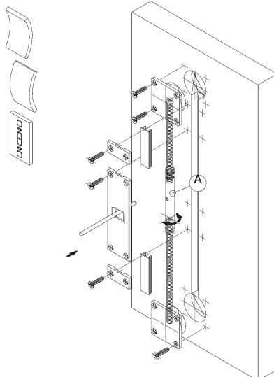
Շտկում A-տեղակայման մանեկի միջոցով
